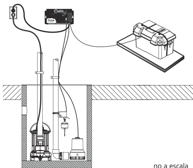
Figura 6. Ejemplo de sistema de bomba de reserva completo
