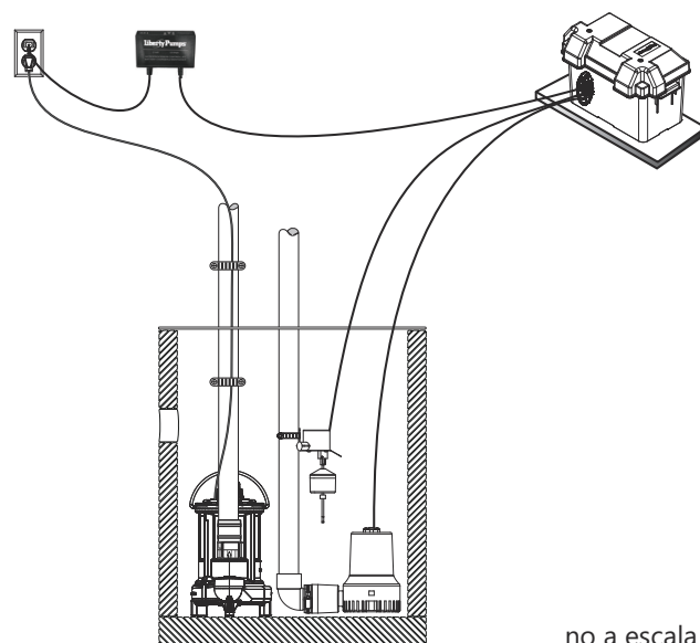
Figura 5. Ejemplo de sistema de bomba de reserva completo
