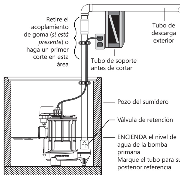
Figura 1. Marcar y cortar el tubo
