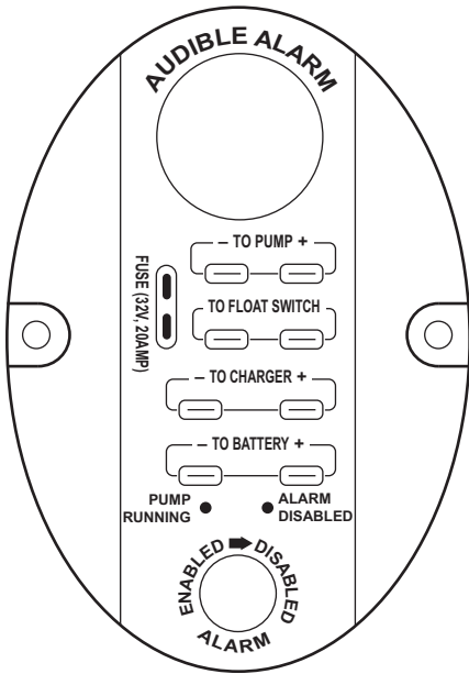
Figura 3. Bloque de terminales
